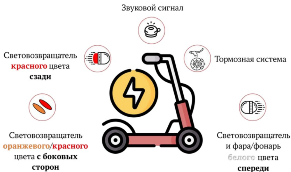
Рисунок 5. Оборудование СИМ
